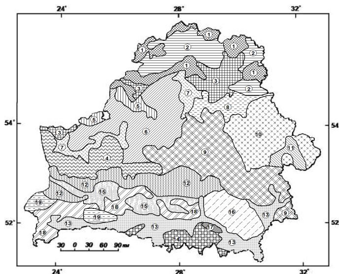
Рисунок 1 - Карта типов инженерно-геологических обстановок территории Беларуси
